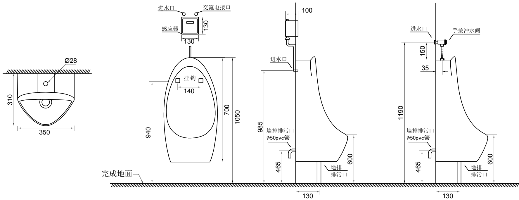
感应器安装示意图
