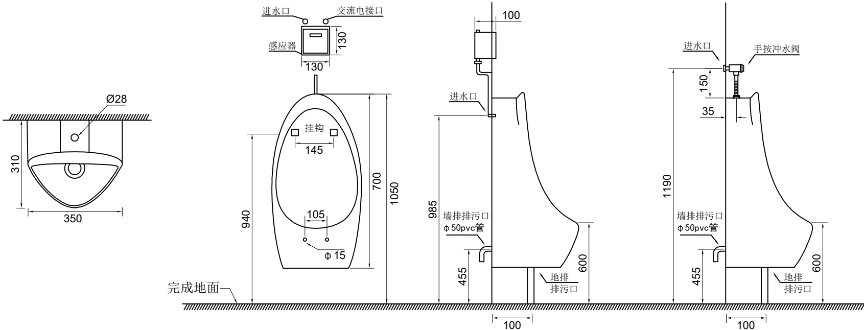
感应器安装示意图
