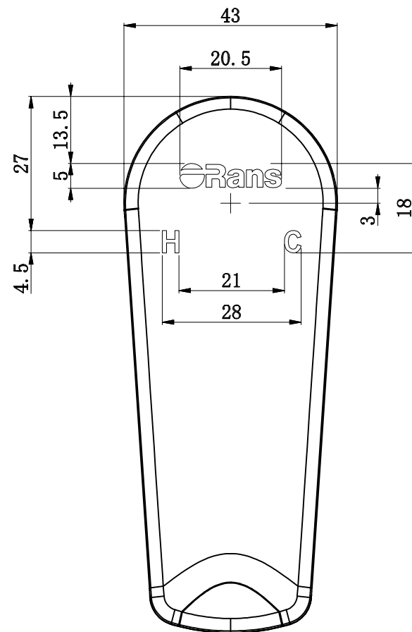
把手 比例 1.000
