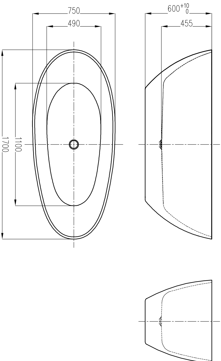
BT-61151B线框图 1700*750*600 (mm)
